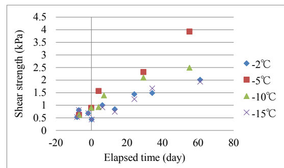
図1 各温度条件における剪断強度の変化
