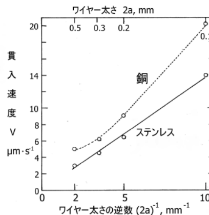
図1 貫入速度 V とワイヤー太さの逆数の関係
