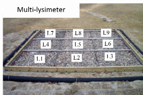
図 1 雪氷防災研究センターに設置された Multi-lysimeter
