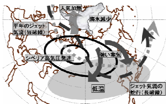
図 2. 北極海の海水減少によって極東一帯に寒波がもたらされるメカニズム。
