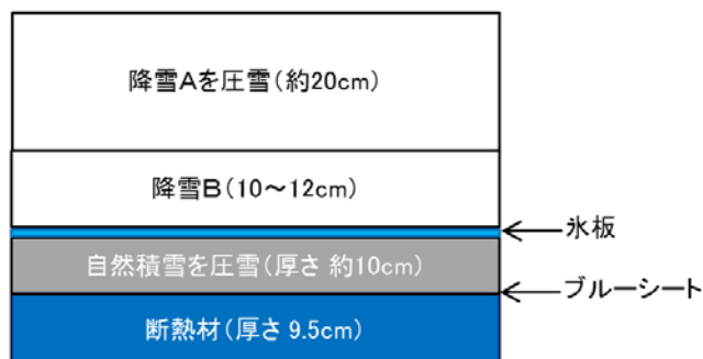
図-1 積雪層の構成(実験前)
