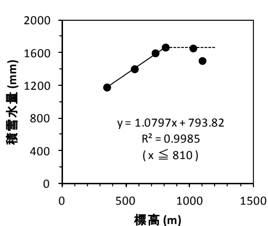
図1 標高と積雪水量の関係。 (2012年2月17日測定)
