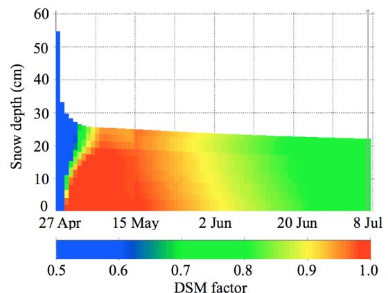
図3 しもざらめ化率の計算例
