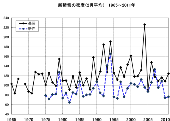
図 2 長岡と新庄の 2 月の新積雪の密度
