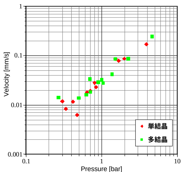
Fig. 1 ワイヤー貫入速度の圧力依存性
