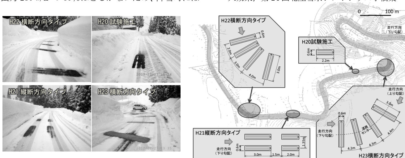
図-1 地熱ヒートパイプ融雪施設の施工位置と施工タイプ
