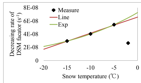
図2 しもざらめ化率の変化の温度依存性
