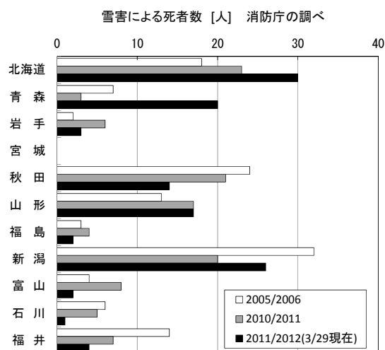
図 3 北海道、東北、北陸の雪害による死者数
