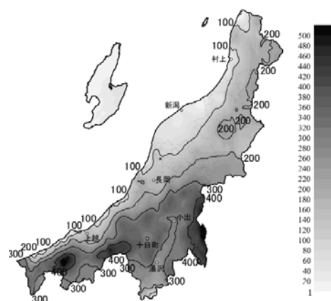
図 2 2011 年 2 月 10 日 9 時の積雪深分布図 (新潟県内 328 地点の Web 公開データを使用)
