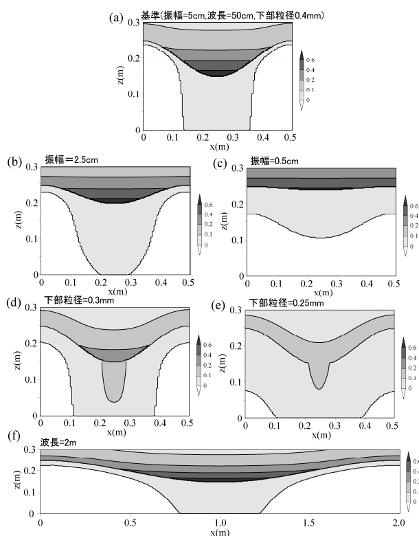
図1 水の供給開始6時間後の体積含水率の分布。 (a)振幅5cm、波長50cm、上部粒径0.2mm、下部粒径0.4mm、(b)振幅2.5cm、(c)振幅0.5cm、 (d)下部粒径0.3mm、(e)下部粒径0.25mm、 (f)波長2m
