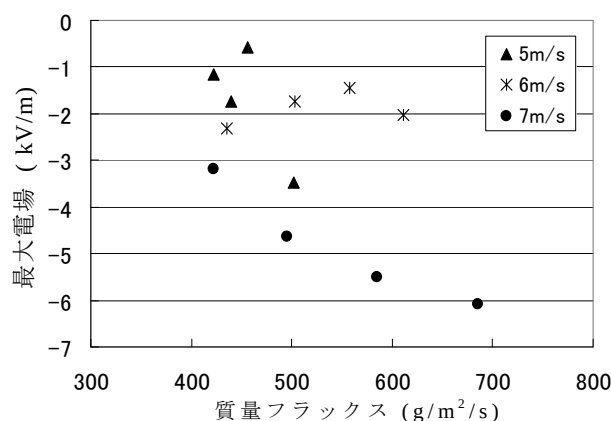
図3 最大電場と質量フラックスの関係
