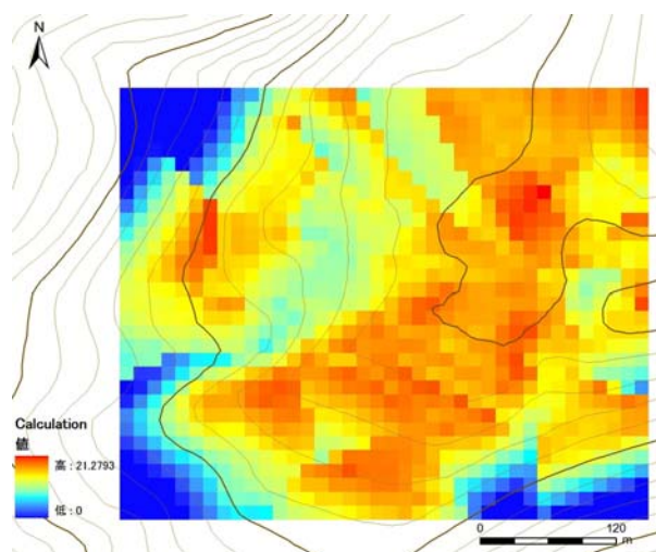
図 2 推定された積雪深分布
