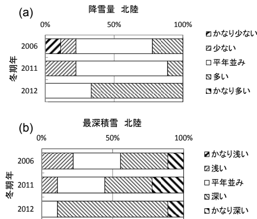
図 2 北陸の冬期間の (a) 降雪量と (b) 最深積雪の階級毎の観測点の割合
