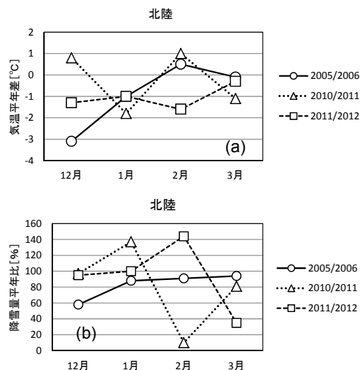
図 1 北陸の (a) 月平均気温の平年差と (b) 月降雪量の平年比
