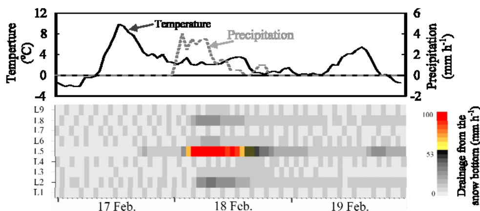
図 2. 2011 年 2/17-19 に観測されたライシメータ間の極端な流出量の違いとその時の気象データ（気温、降水量）
