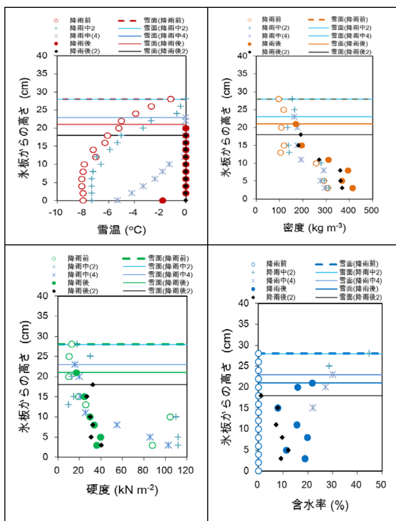
図-2 実験中の雪温、密度、硬度、重量含水率の変化
