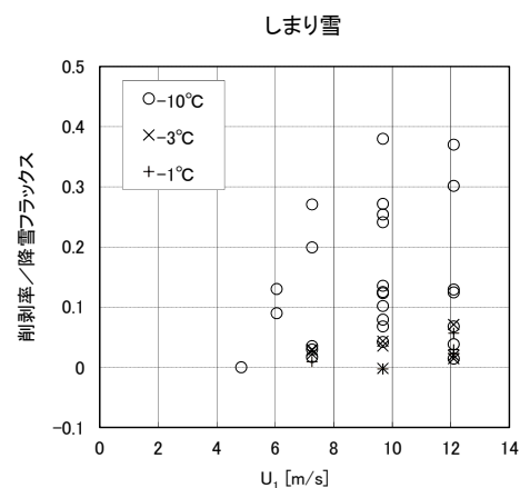
図2 降雪フラックスで規格化した削剥率と風速の関係。積雪面はほぐしたしまり雪で、気温を変えた。
