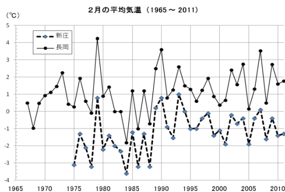
図 1 長岡と新庄の 2 月の平均気温
