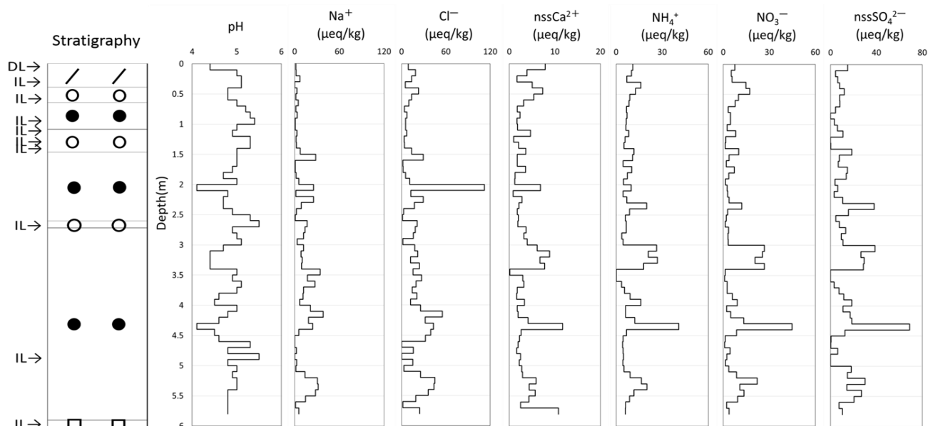
図 1 立山・室堂平（2017 年 4 月）における積雪層位およびイオン成分濃度の鉛直プロファイル
