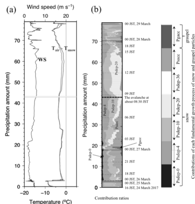
図1 那須町雪崩地点を含むモデル格子の気象パラメータを、2017年3月24日1600JST以降の10分毎積算降水量積算降水量の関数として表記した層位図。(a)地上風速(WS), 気温( T_{\text{air}} ), 雪温( T_{\text{snow}} )。 (b)素過程別成長量の寄与率毎に色分けしたもの。PdepXは温度別昇華生長量(Pdep-0: 0~-4°C, Pdep-4: -4~-10°C, Pdep-10: -10~-20°C, Pdep-20: -20~-36°C, Pdep-36: -36°C以下), Psacc: 雪の雲粒捕捉生長量, Pgacc: 霰の雲粒成長量。(橋本ほか, 2017, 雪氷研究大会講演予稿集, p73)
