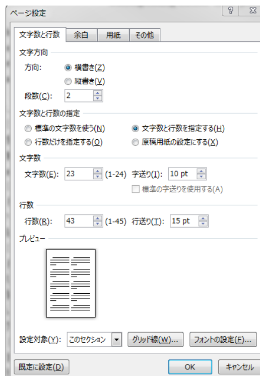
図1 ページ設定
