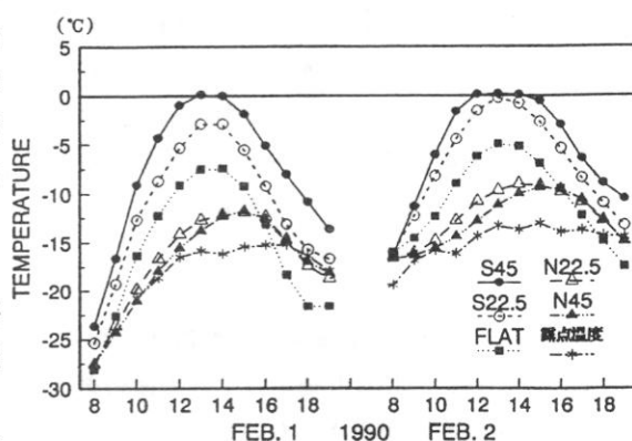
図2. 斜面の表面温度および露点温度 (1990年2月1日、2日)
