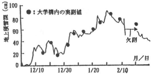
図2 地上積雪深の推移
