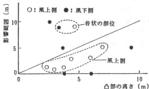
図8 凸部の高さで影響範囲との関係
