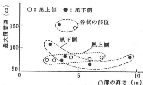
図6 凸部の高さで最大積雪深との関係
