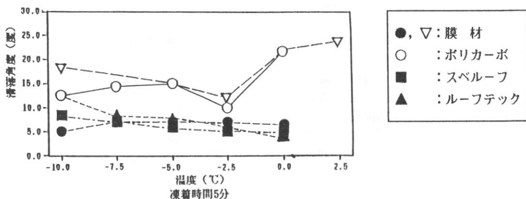
図3 温度と滑落角度の関係
