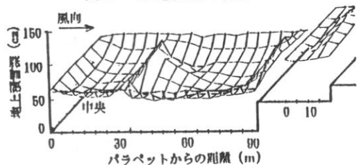
図3 屋上積雪分布の一例(2号館屋上)
