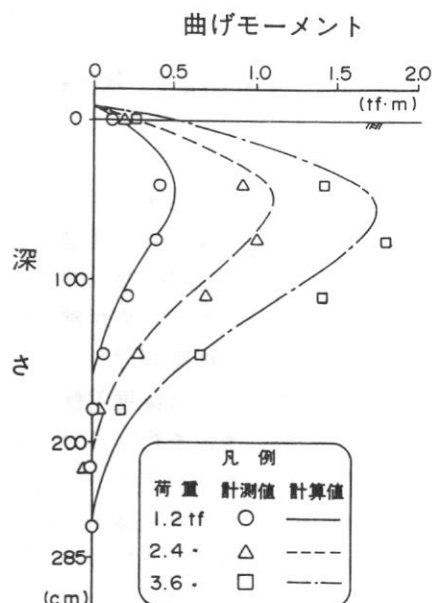
図-3 曲げモーメント分布の計算値と計測値を比較
