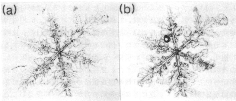
図3 雪結晶のレプリカ作製例：(a)レプリカ前 (b)できたレプリカ。 ポリスチレンの1,1,1-トリクロロエタン10%溶液使用。雪結晶の直径約4mm。
