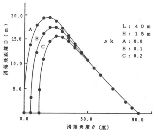
図5 滑落角度と滑落飛距離の関係
