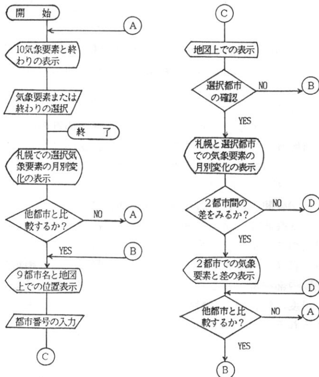
図1 CAIソフト“札幌の気候”フローチャート
