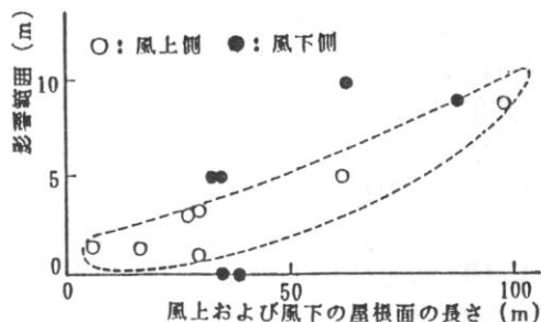
図9 風上屋根面長さで影響範囲との関係
