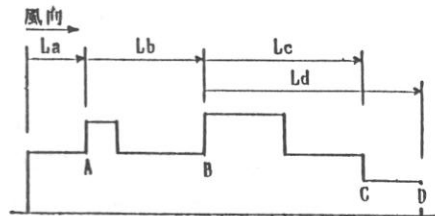
凡例) La: A点に影響を及ぼす屋根面の長さ 図4 影響を及ぼす屋根面長さの定義
