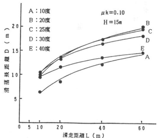
図6 滑走距離と滑落飛距離の関係
