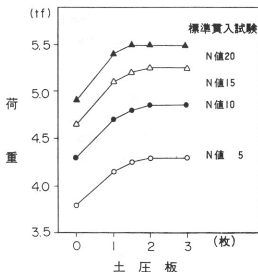
図-4 土圧板の設置効果
