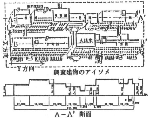
図1 調査対象建物の概要
