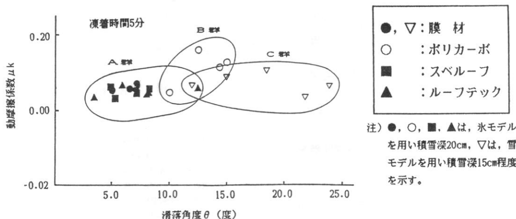
図4 滑落角度と動摩擦係数の関係
