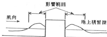
図5 影響範囲の定義
