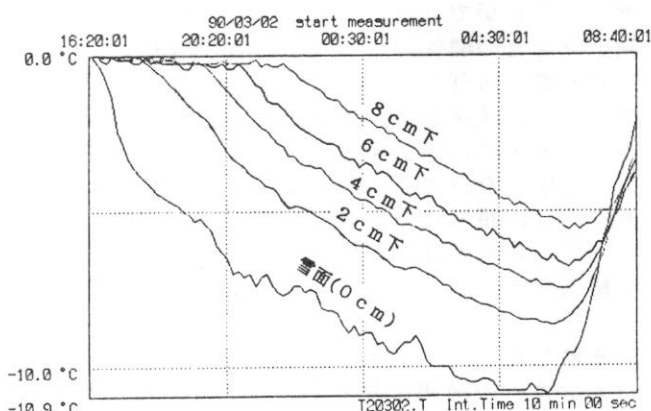
図2 各深さでの雪温の時間変化(3/2~3)
