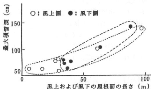
図7 風上屋根面長さで最大積雪深との関係
