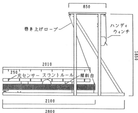
図1 滑落装置
