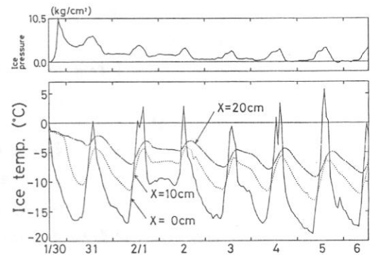
図-2 屈斜路湖における実測値と熱応力
