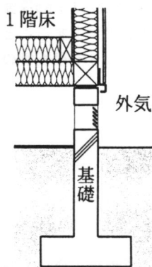
図 1-1 床断熱工法
