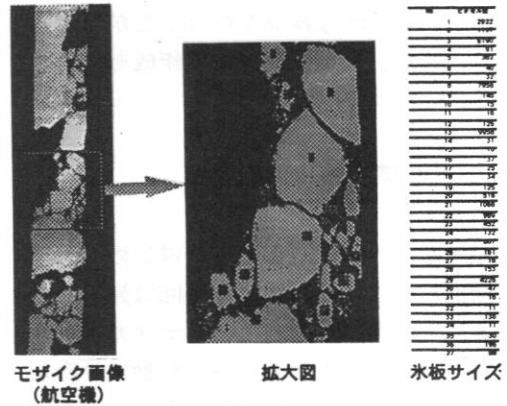
図3 モザイク画像より求めた氷板サイズ
