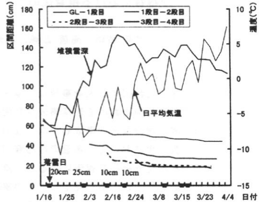
図 6 軒下から 150cm 地点の区間距離と最大堆積雪新および平均温度
