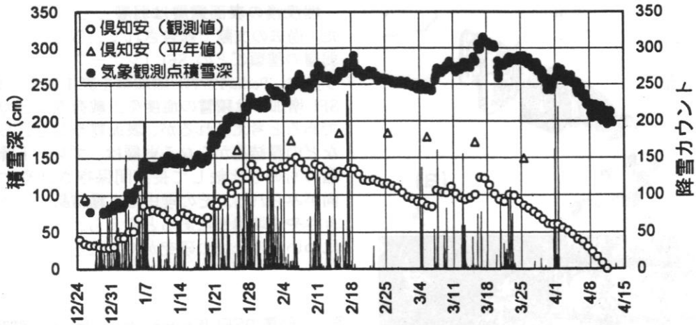
図2 積雪深と降雪カウント数の時系列変化
