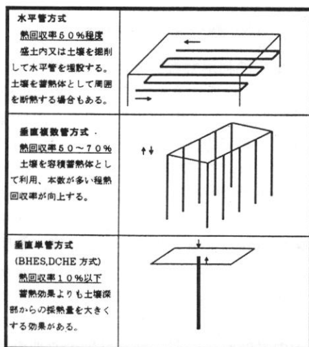
図-2 3方式の地中熱交換器モデル
