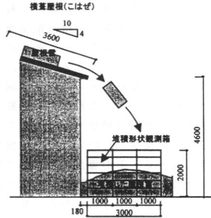
図2 試験体寸法図
