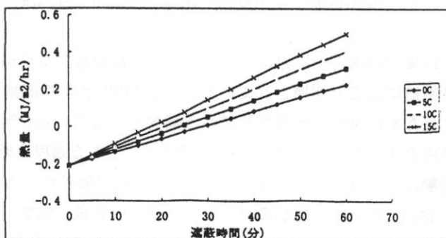
図2. 車に遮蔽された道路積雪面の総熱量
