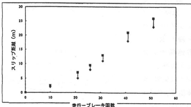
図3. ブレーキ回数と制動距離の関係
