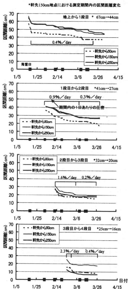
図5 軒下堆積雪の層内圧密の状況
