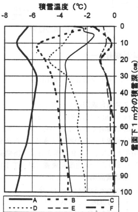
図6 積雪温度の鉛直プロファイル
