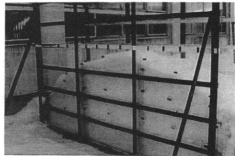
写真4 堆積雪断面の沈降量測定
