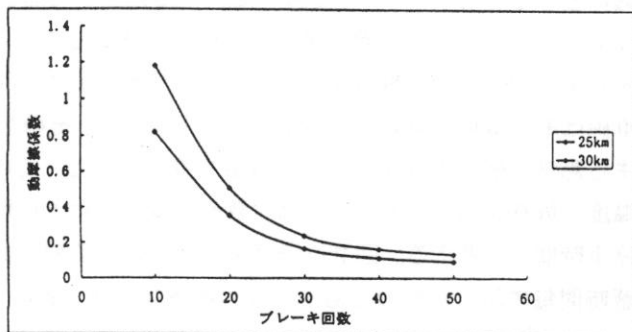
図4. 制動試験による道路積雪面の摩擦係数の変化
