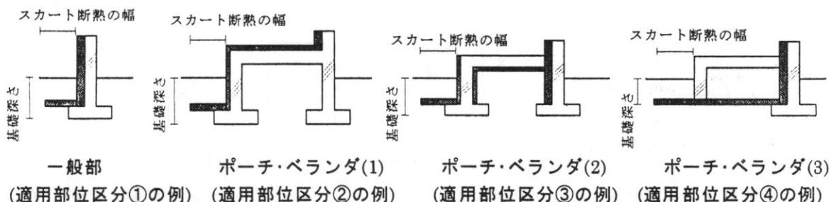
図 6 適用部位区分①～④に分類される基礎の各部位・仕様の例
