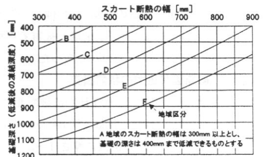
図 7 幅決定用グラフ (適用部位区分②)
