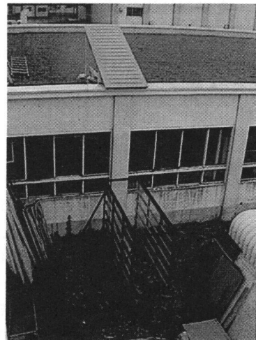
写真3 屋根と堆積形状観測箱
