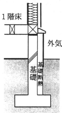
図 1-2 基礎断熱工法
