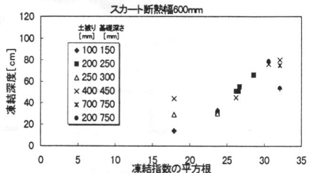
図4 凍結指数の平方根と凍結深度の関係 (スカート断熱幅 600 mm の例)
