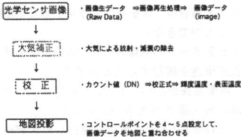
図3 光学センサデータの処理
