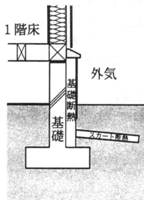
図 1-3 スカート断熱工法
