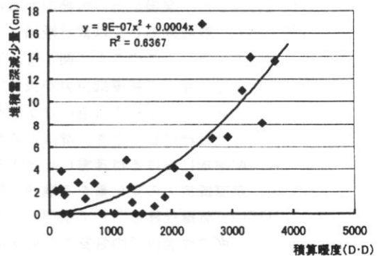
図 7 融雪期における堆積雪深減少量と積算暖度
