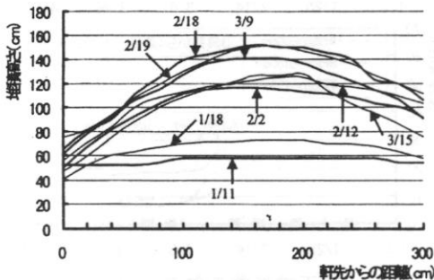
図3 滑落後の軒下堆積雪形状
