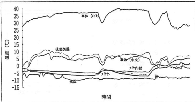
図1. 気温・車体各部の温度(29日10-12時)
