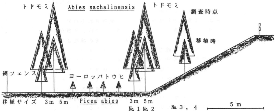
図-1 トドモミの成木移植地の横断模式図（N27KPふきん）
