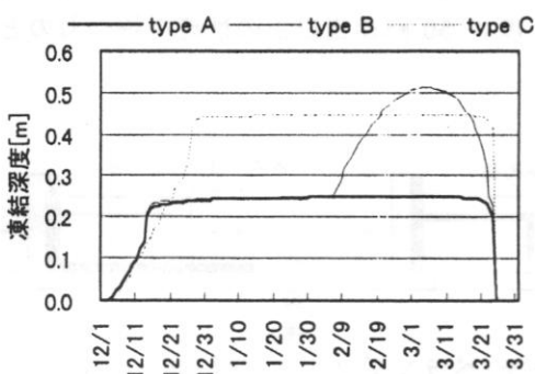
図3 基礎コーナー部分の凍結深度計算結果
