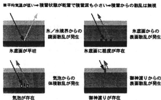
図5 屈斜路湖のマイクロ波散乱機構
