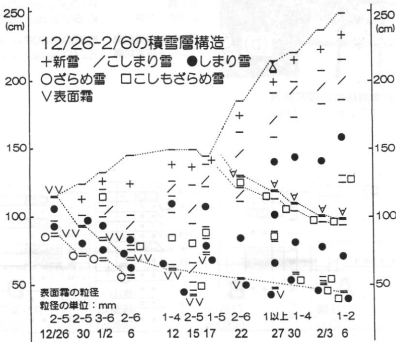
図3 積雪層構造の時系列変化
