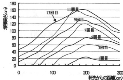
図4 連続的に滑落させたときの形状
