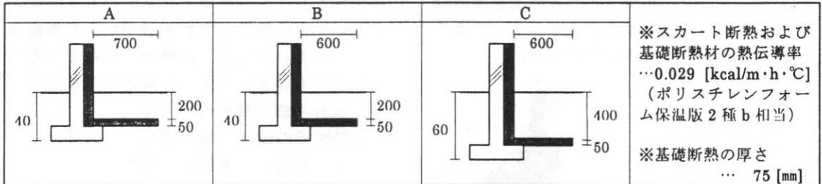
図2 シミュレーションのモデル (A・B・C)
