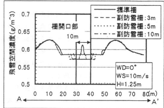
図 3. 2 縦断方向の飛雪空間濃度分布
