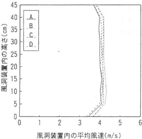
図2 実験時の風洞内風速分布
