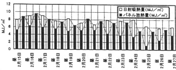
図 4 (a) パネル表面加熱量変化 (黒色) 昼間夜間に分けた日出没時までの積算量
