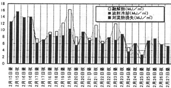
図 5 (a) パネル表面熱損失量変化 (黒色) 昼間夜間に分けた日出没時までの積算量
