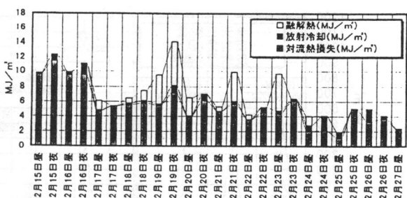
図 5 (b) パネル表面熱損失量変化 (灰色) 昼間夜間に分けた日出没時までの積算量
