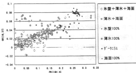
図 3. 分類 [PR (18V, H) - GR (18, 37)]
