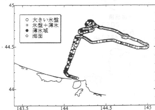
図 4. AMR の航跡上の海氷分類図
