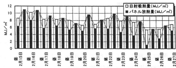
図 4 (b) パネル表面加熱量変化 (灰色) 昼間夜間に分けた日出没時までの積算量
